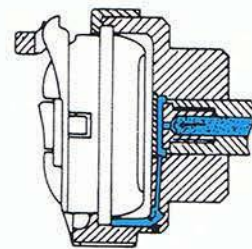
Full-automatic system-open type 自动润滑开放型
