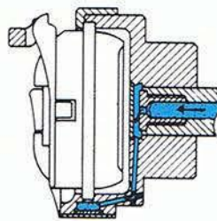
Full-automatic system-closed type 自动润滑封闭型
