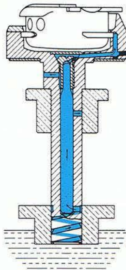
Full-automatic system vertical axis hook 水平梭头 I 型
